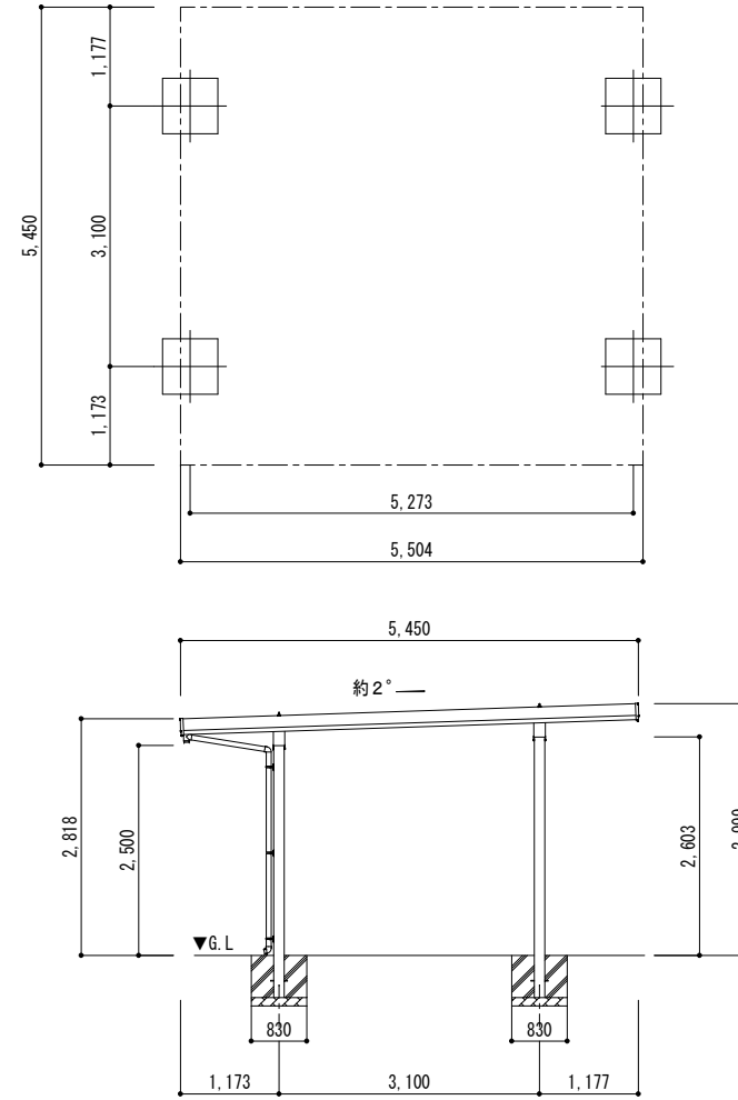
■基礎配置図
