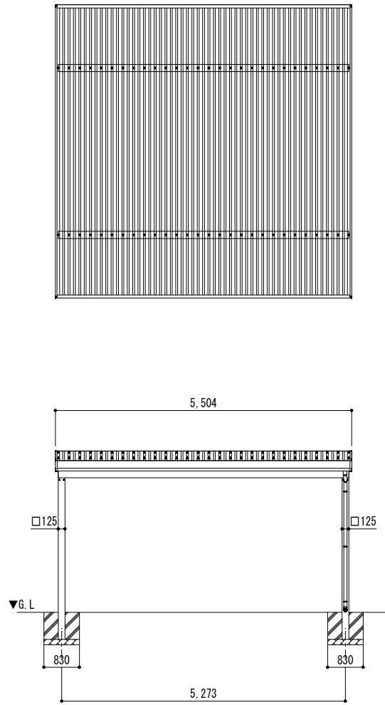
■姿図
